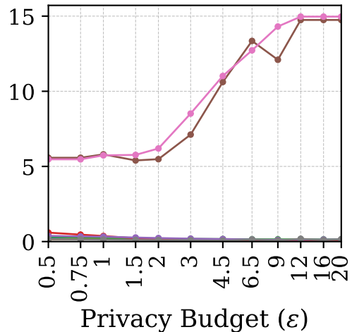
Brightkite
